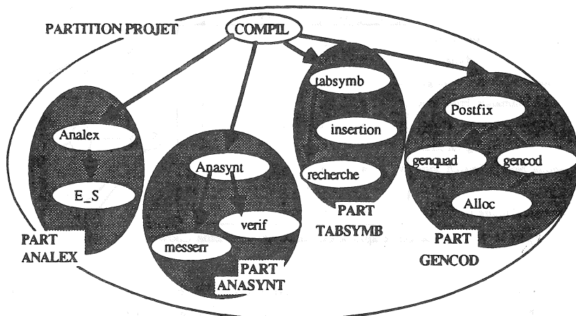
Figura 5 - Ejemplo de estructuración de software en Adèle
